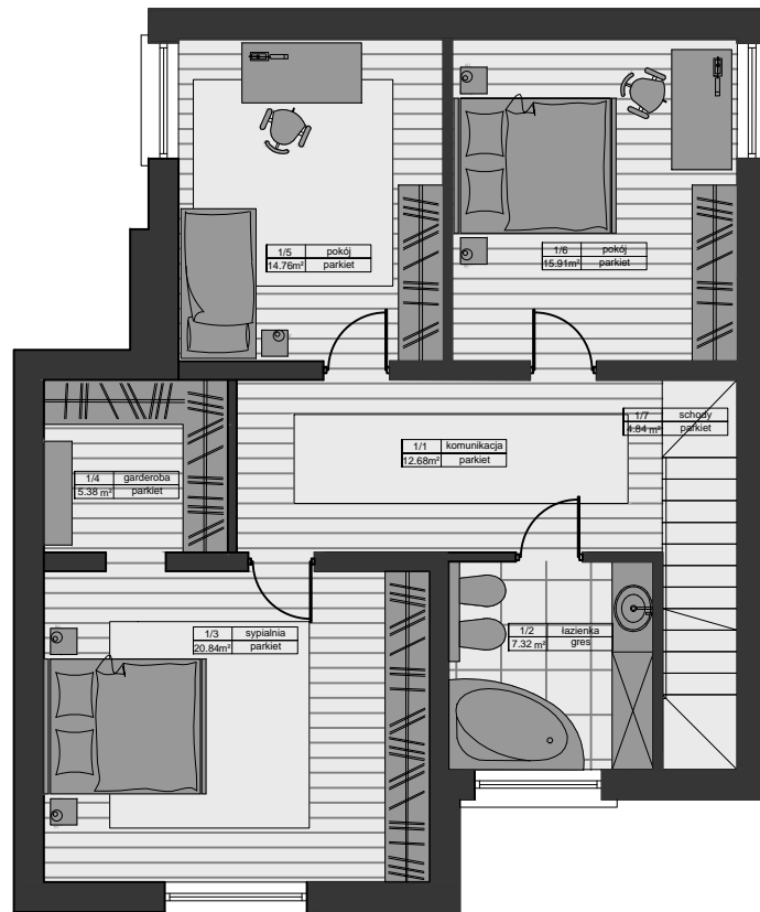
PIĘTRO
